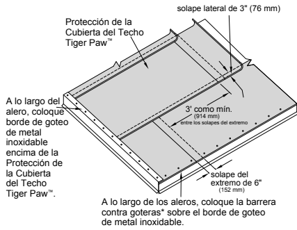
Figura 1 – Aplicación Estándar Para Pendiente De 4:12 O Más
