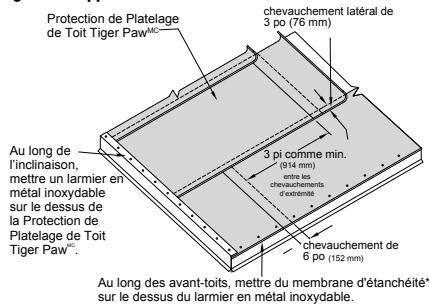
Figure 1 – Application Standard Pour Des Pentes De 4:12 Ou Plus
